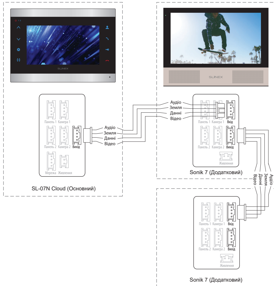
Схема 2. Підключення системи домофонів SL-07N Cloud і Sonik 7
